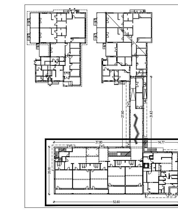
TLORIS PRITLIČJA - osnovni del M 1:50
